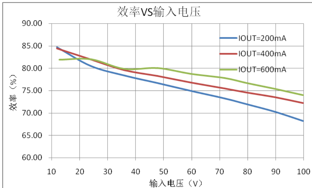
(2) 输出 5V/0.6A 输出与输入电压特性曲线
