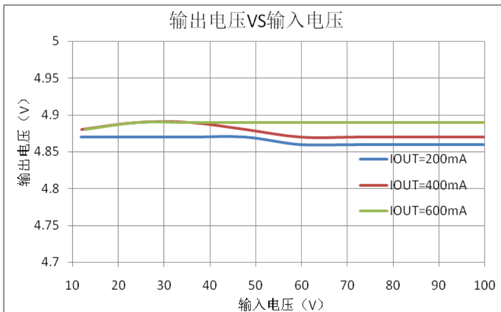
(2) 输出 5V/0.6A 输出与输入电压特性曲线
