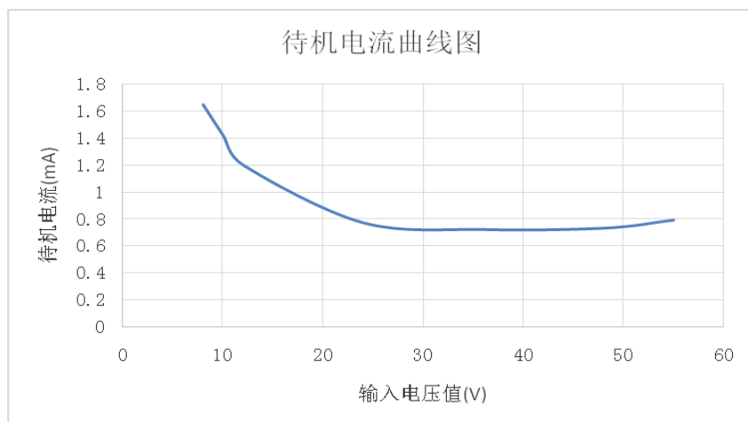
待机电流与输入电压特性曲线
