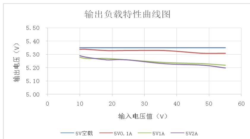
输出负载与输入电压及输出电流特性曲线 (V0=5V)
