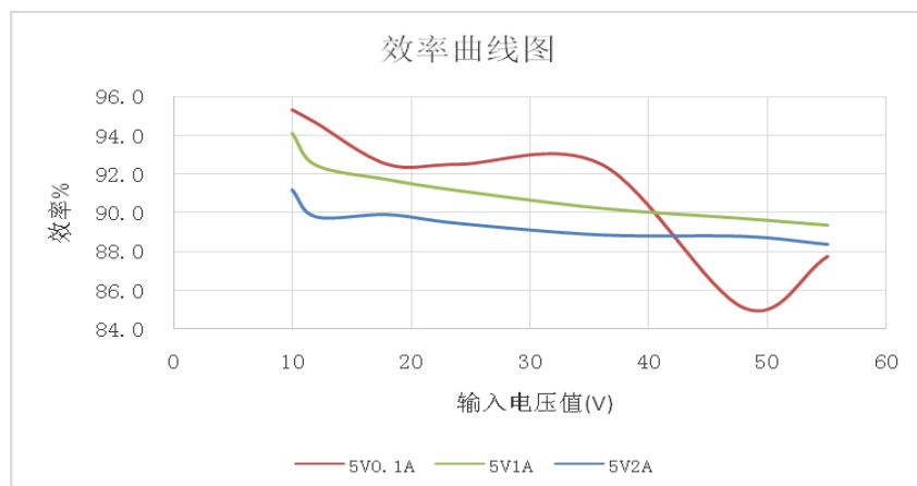
效率与输入电压及输出电流特性曲线 (V0=5V)
