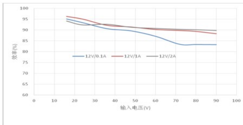
(2) V_O=5V/2A 效率与输入电压特性曲线
