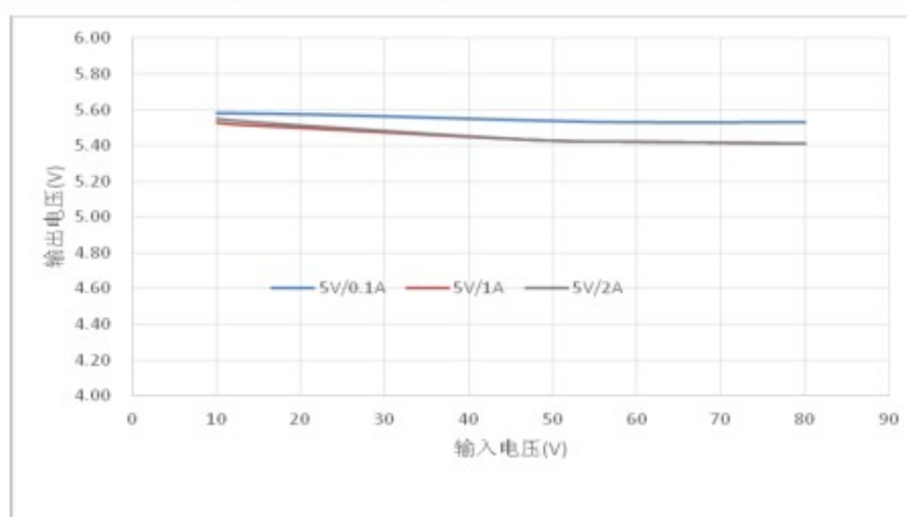
(3) V_O=5V/2A 输出电压与输入电压特性曲线
