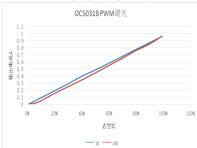
PWM 调光特性曲线
